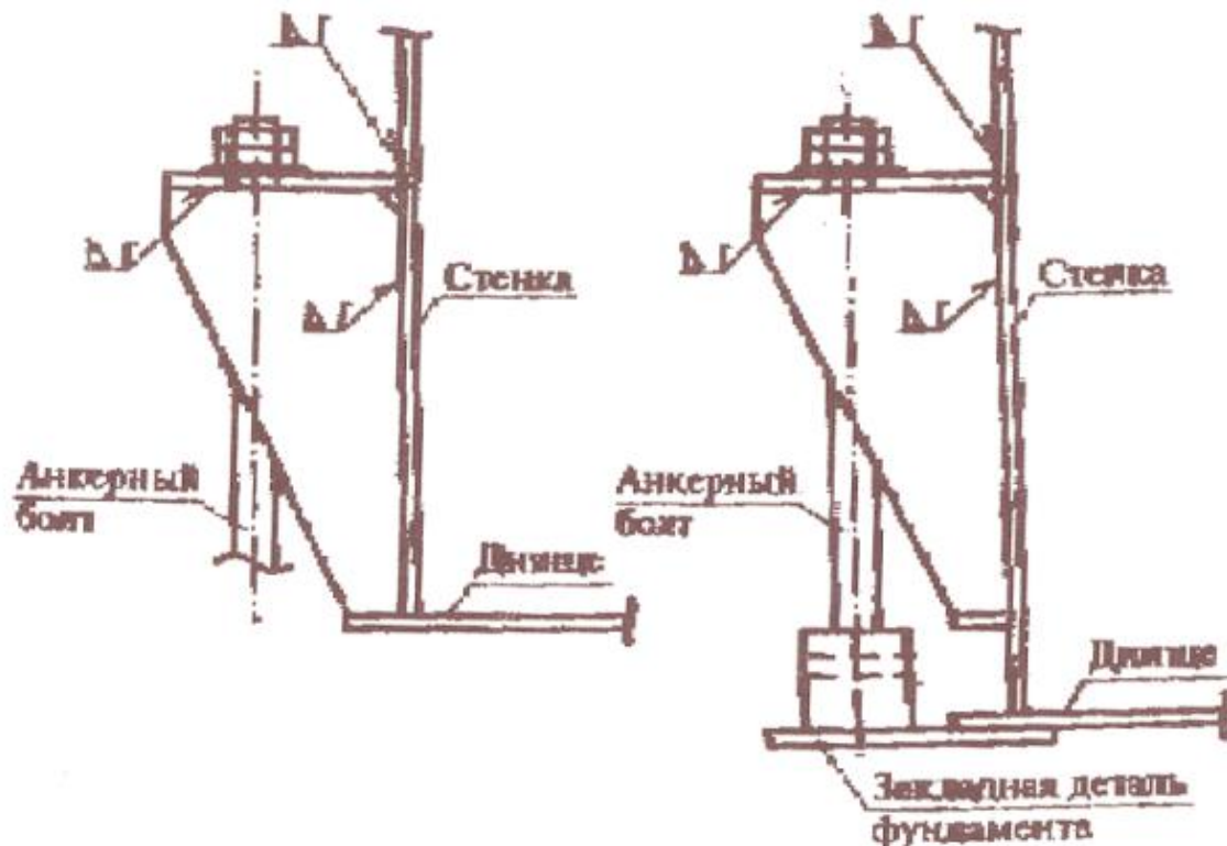
Рис. 3.16. Анкерное крепление стенки.
