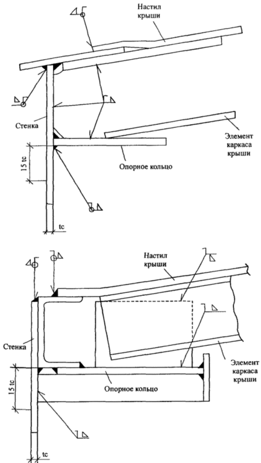
Рис. 3.8. Соединение сферической крыши со стенкой.
