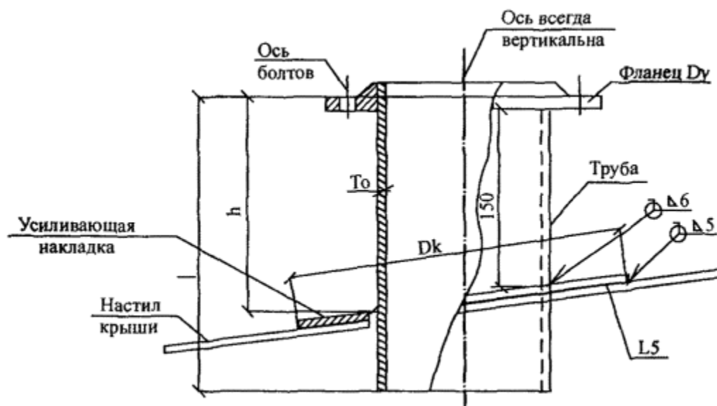
Рис. 3.14. Патрубки на крыше.
