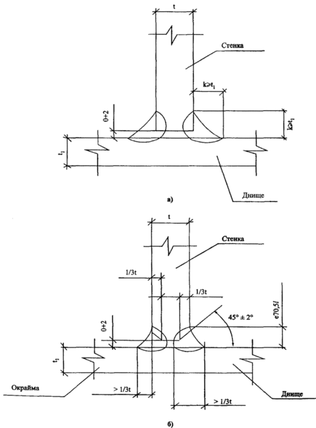
Рис. 3.6. Соединение днища со стенкой.
