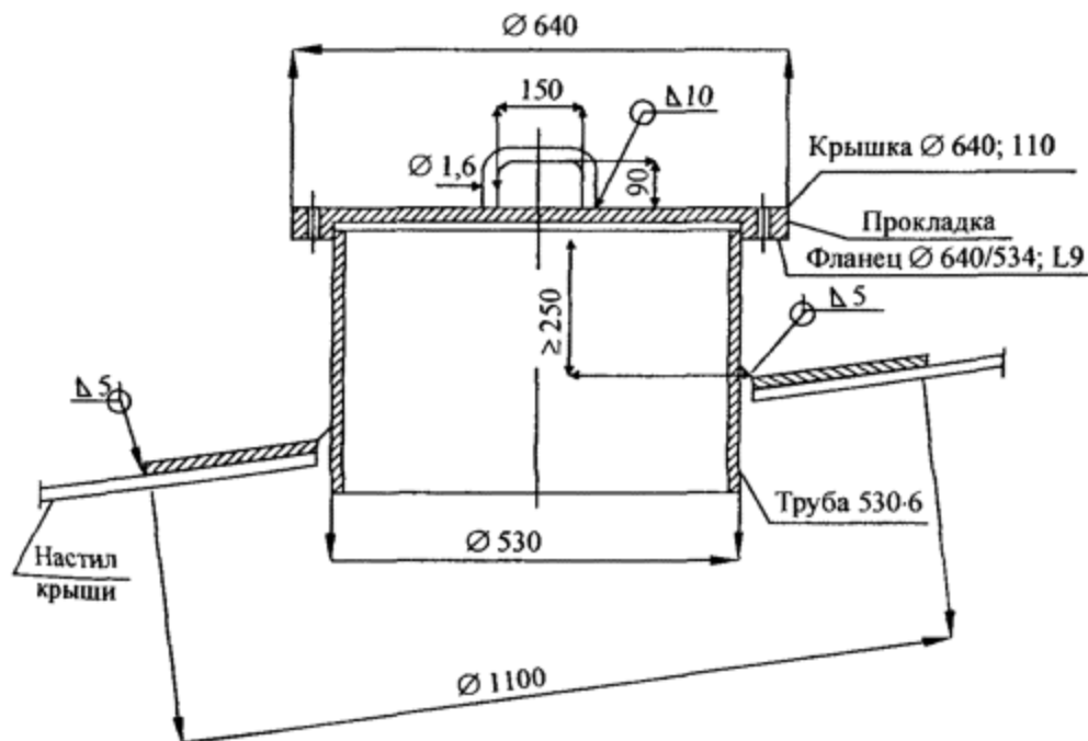
Рис. 3.15. Люк световой D_y 500.
