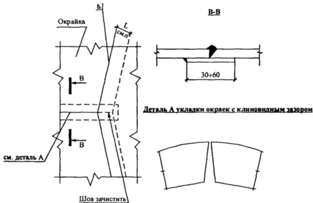
Рис. 3.5. Соединение центральной части с окрайками днища.
