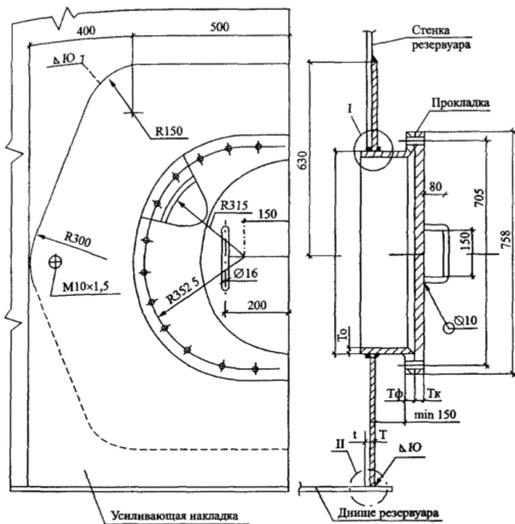
Рис. 3.10. Люк-лаз круглый в I поясе стенки.
