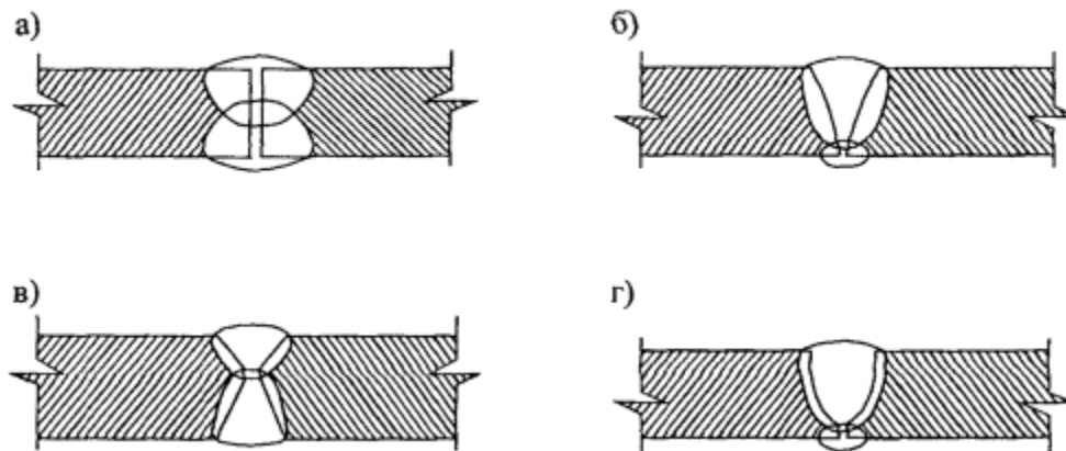
Рис. 3.1. Вертикальные стыковые соединения стенки:
