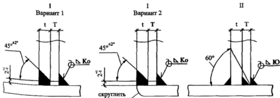
Рис. 3.11. Люк-лаз овальный 600×900 мм в I поясе стенки.
